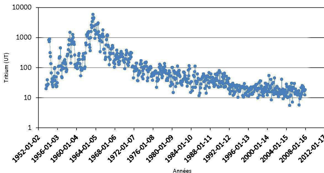
Figure 5.29: Tritium dans les précipitations Ottawa (1953 à 2007) selon les données de l'AIEA (IAEA/WMO, 2012).
